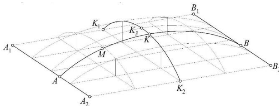
6-rasm. Ikki egri chiziqli qobiq sirtini modellashtirishning geometrik sxemasi.
