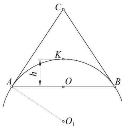
2-rasm. Doira yoyining muhandislik diskriminanti qiymatini aniqlashning geometrik sxemasi.
